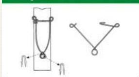
Distanziatore mobile di fili doppi con fissaggio al palo di legno tramite cambrette
